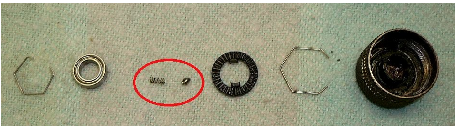
Teile des Spulenfreilaufs. Bei der Wartung unbedingt auf den winzigen Ratschenpin achten!!!
