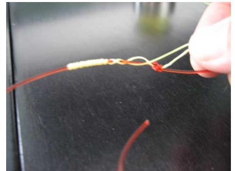
Bild 6 Zuerst die 8 kräftig zuziehen. Dann die Braid mit ordentlichem Zug auf beiden Enden an die 8 heranziehen, Man kann dabei auch sanft ein wenig anschieben, aber Schritt für Schritt immer dichter ziehen. Zum Schluss mit vollem Zug an den Braidenden den Knoten zum Sitzen bringen.
