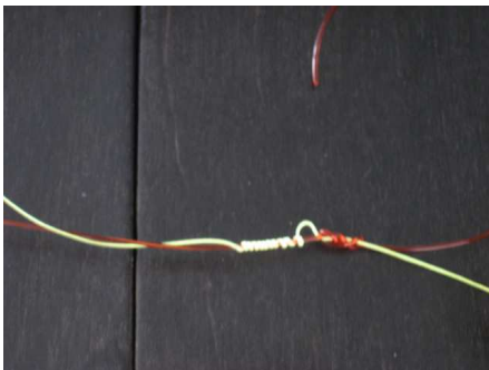
Bild 4 Das Detail nochmals etwas näher fotografiert.
