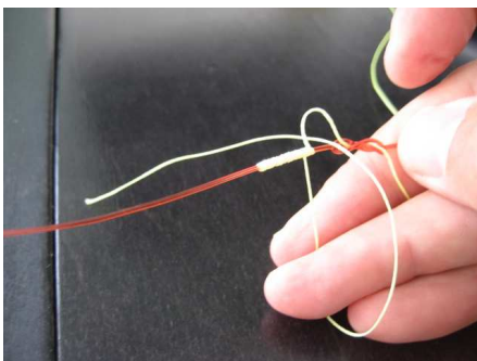
Bild 5 Nun mit der Braid erneut 10-15 Wicklungen auf den bereits liegenden Wicklungen zurück zur kleinen Schlaufe bei der 8 fahren. Alles schön mit leichtem Zug. Nun wird das Braidende wie auf dem Bild zu sehen durch die Schlaufe geführt.
